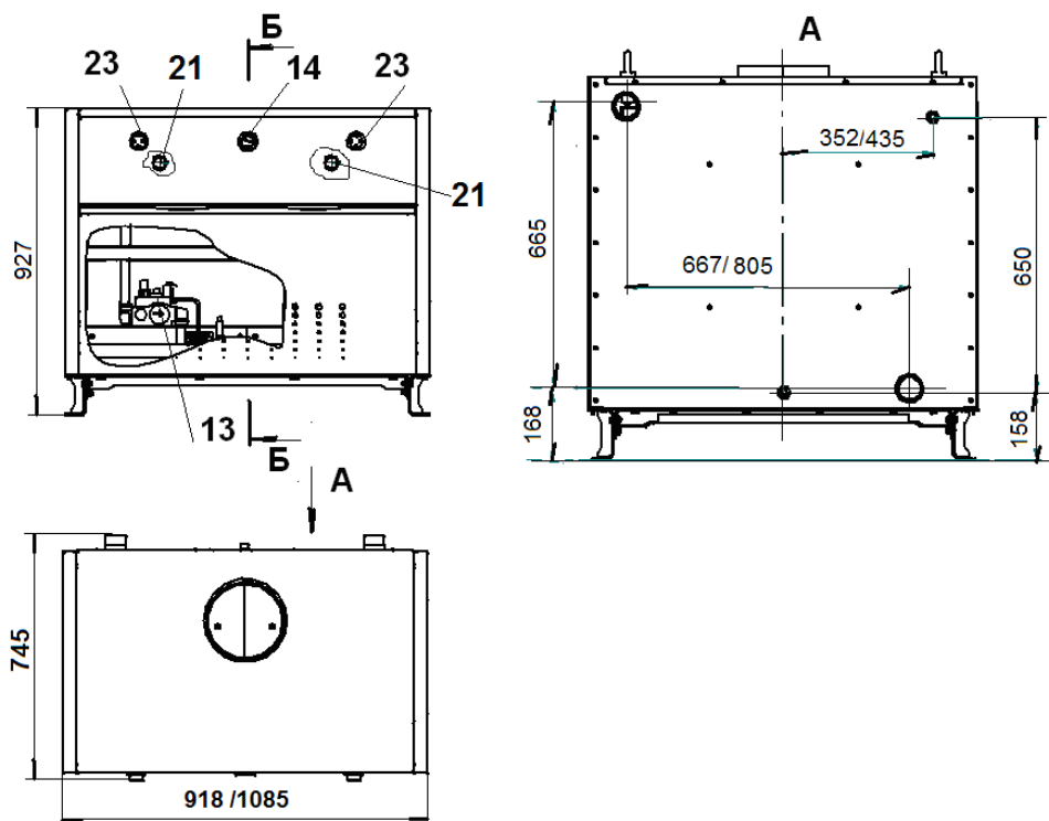
Рис. 2 Котлы КС-Г-80S-1 и КС-Г-100S-1 Остальное см. рис.1
